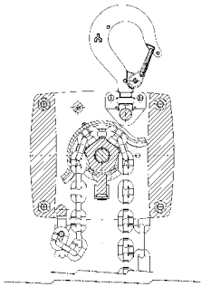
Yalelift 0,5 - 3 t
